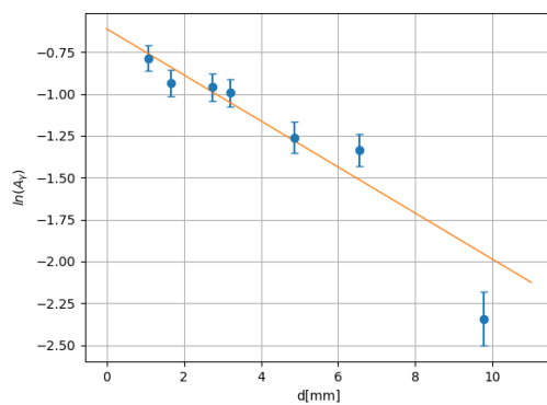
Slika 3: Graf \ln(A_\gamma)(s) za svinec
